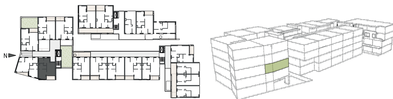
GEBOUW A / NIVEAU 2 / APPARTEMENT A2.5 / 64 m²
