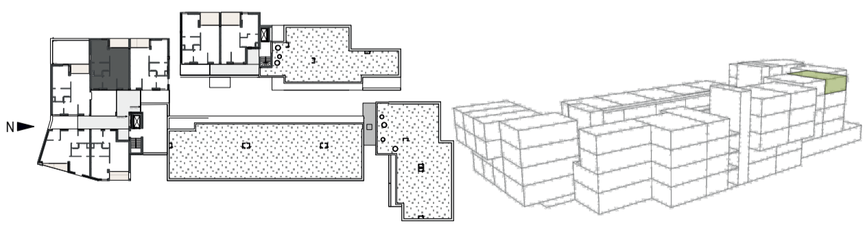
GEBOUW A / NIVEAU 4 / APPARTEMENT A4.2 / 69 m 2
