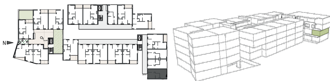
GEBOUW C / NIVEAU 1 / APPARTEMENT C1.9 / 52 m 2
