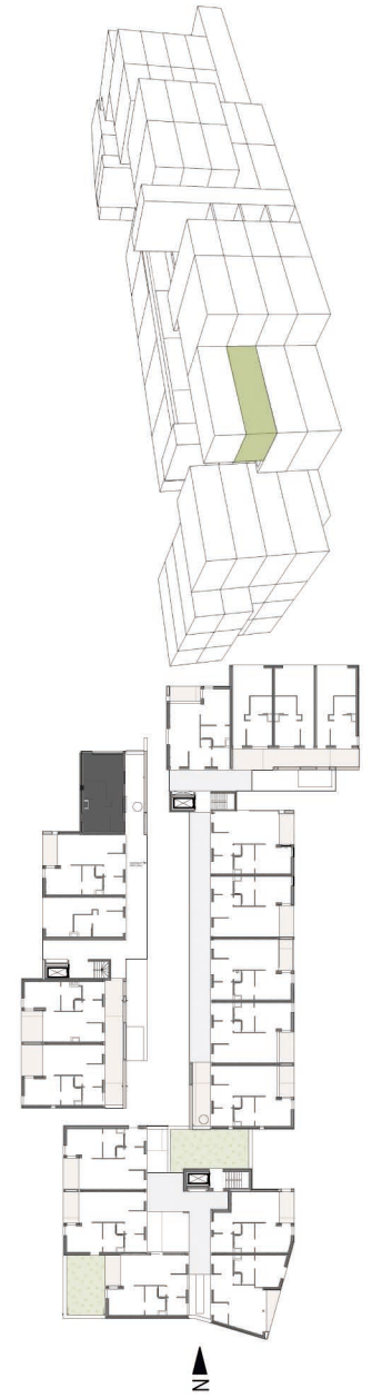
GEBOUW B - NIVO 2 - APPARTEMENT B2.5 - 53 m 2
