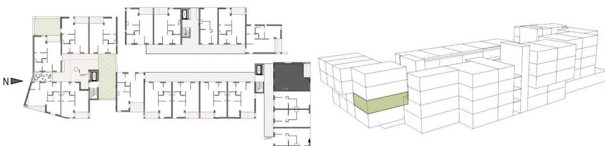
GEBOUW C - NIVO 1 - APPARTEMENT C1.6 - 70 m 2
